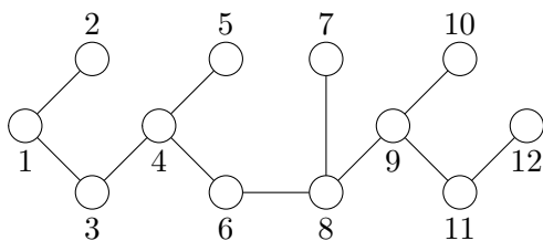
Beispiel 28 (Tiefensuche):
