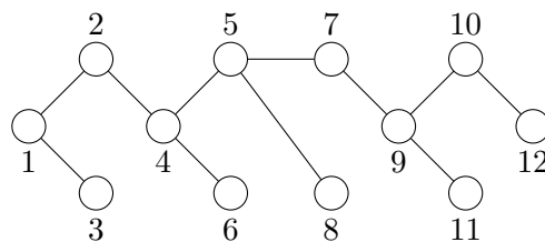
Beispiel 29 (Breitensuche):
