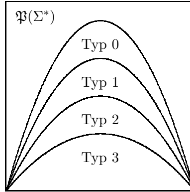
Abbildung 3.1.: Chomsky-Hierarchie
