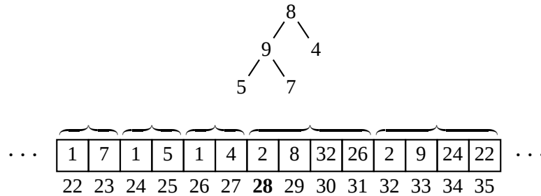
Abbildung 15.1: Darstellung eines Baums in der Halde
