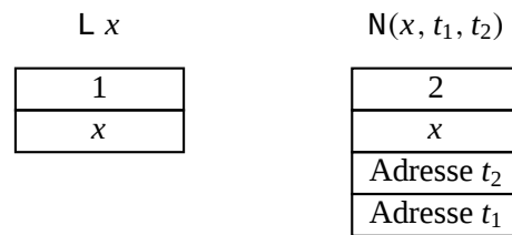
Abbildung 15.1: Darstellung eines Baums in der Halde
