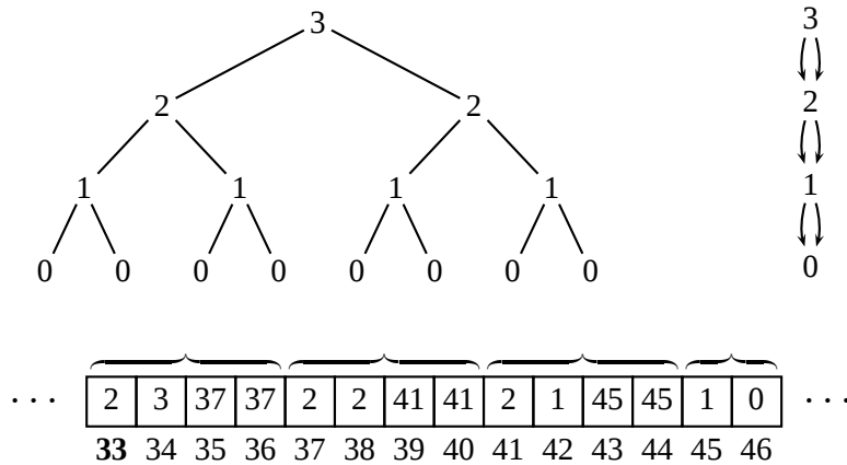
Abbildung 15.2: Darstellung eines Baums durch eine Graphstruktur
